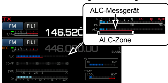
Multifunktionsmessgerät
